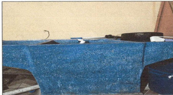
Foto 3: Sustitución de pila de cemento de dos lavaderos
